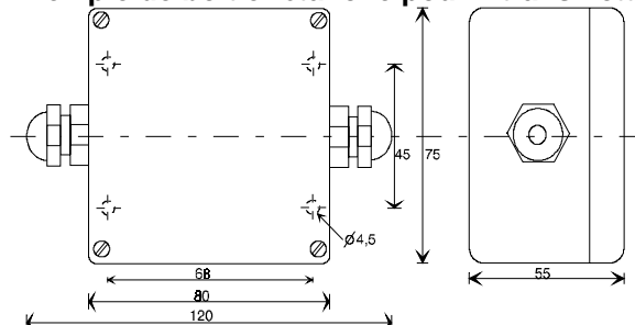
XT4*SI.-BCL Boîtier IP65 polyester chargé
